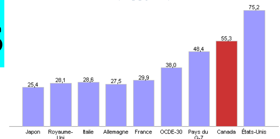
Consommation d'énergie reliée aux transports par habitant, transport routier, pays du G7 et moyenne des 30 pays membres de l'OCDE, 2004 (en gigajoules)
